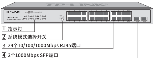
图1-2 TL-NS620-24G2F前面板示意图
